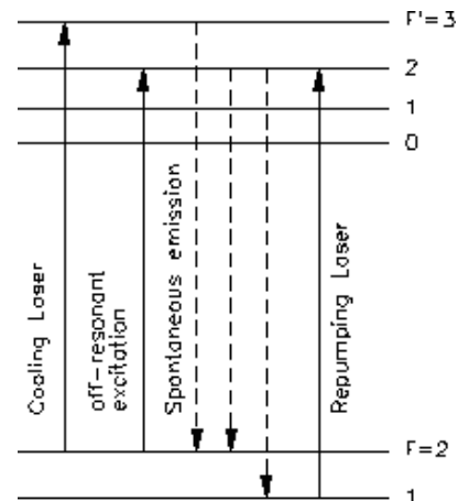
(b) Der Kühllaser treibt den Übergang F = 2 \rightarrow F' = 3
