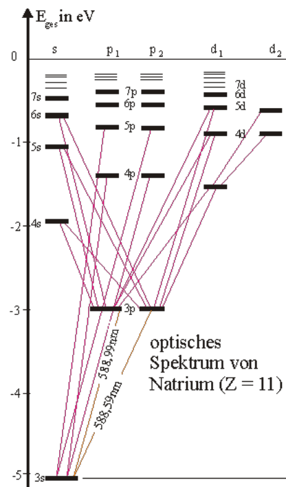
Abbildung 3: Niveauschema des Natrium-Valenzelektrons
