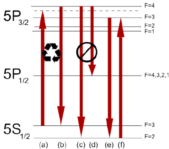
Abbildung 7: Laserübergänge, die für das magneto-optische Festhalten von Rubidium ^{85}\text{Rb} gebraucht werden. a) und b) zeigen den Absorptions-Emissionszyklus. Die Laserfrequenz ist bis zur gestrichelten Linie im Energiediagramm rotverstimmt. c) und d) sind aufgrund von Auswahlregeln verbotene Übergänge. e) zeigt die Möglichkeit, dass ein angeregtes Atom aus dem F = 3 -Zustand in den für den Kühllaser "blinden", tiefliegenden F = 2 -Hyperfeinzustand zerfällt. Dieser Effekt würde sowohl den Kühlvorgang abbrechen, als auch die Fallen-Wirkung aufheben, wäre da nicht der Rückpump Laser f). [Wikipedia - Magneto-Optical Trap]
