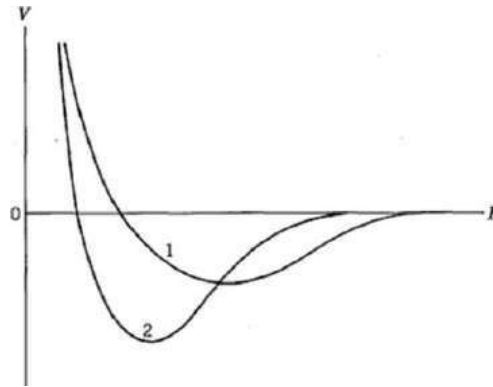
Abbildung 2: Potentialverlauf im Molekül als Funktion des Kernabstands R . Ent stammt „Quantum Physics“ von Eisberg und Resnick, Kap. 12, S. 439.
